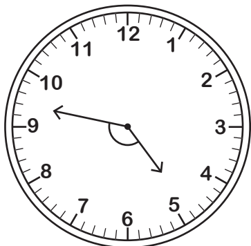
Obtuse angle
