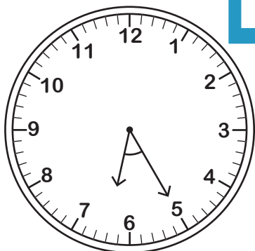
Acute angle
