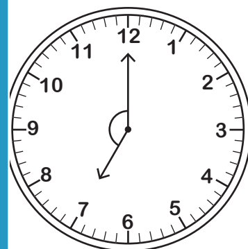
Obtuse angle
