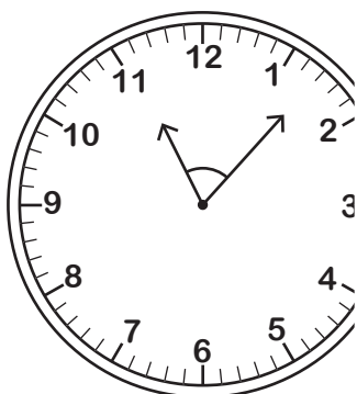
Acute angle
