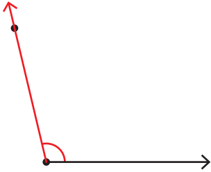
Obtuse angle
