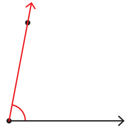
Acute angle
