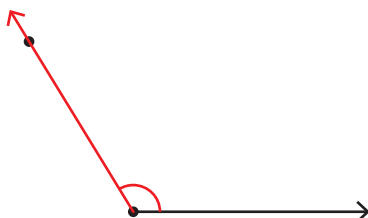
Obtuse angle
