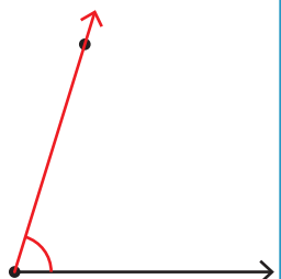
Acute angle
