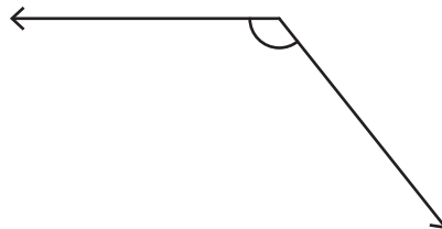
Obtuse angle
