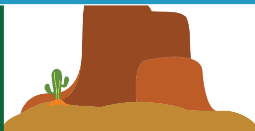
mesa
