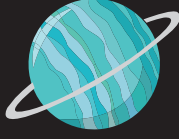
Uranus
