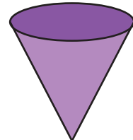
Cone
