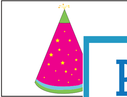
cone
